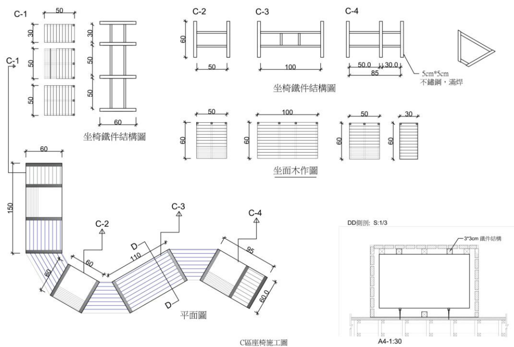
C 區座椅施工圖
