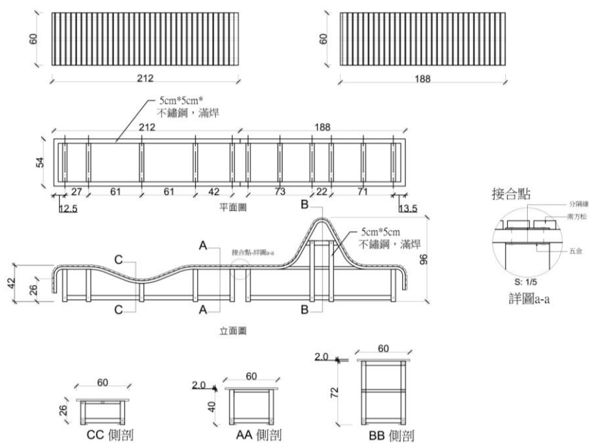
A-3座椅施工圖
