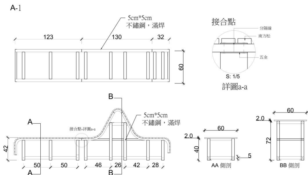
A-1 座椅施工圖
