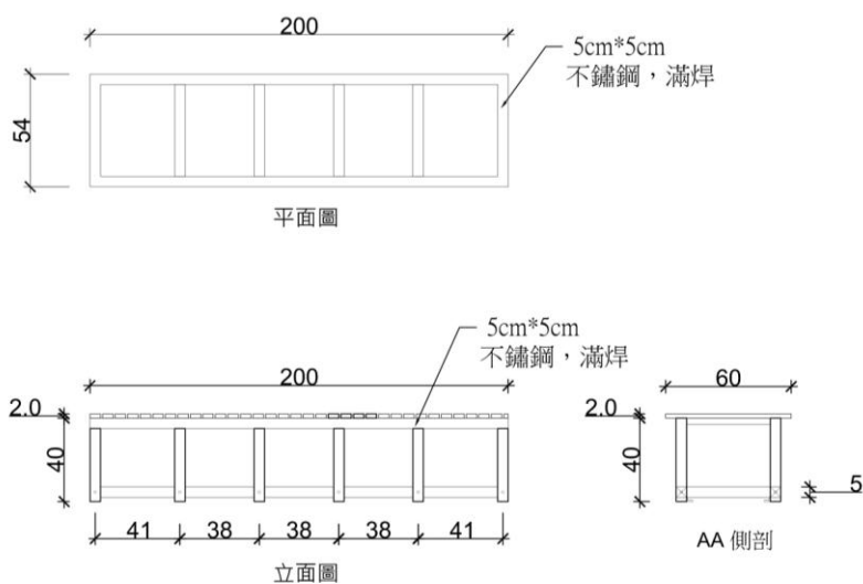
A-2 座椅施工圖
