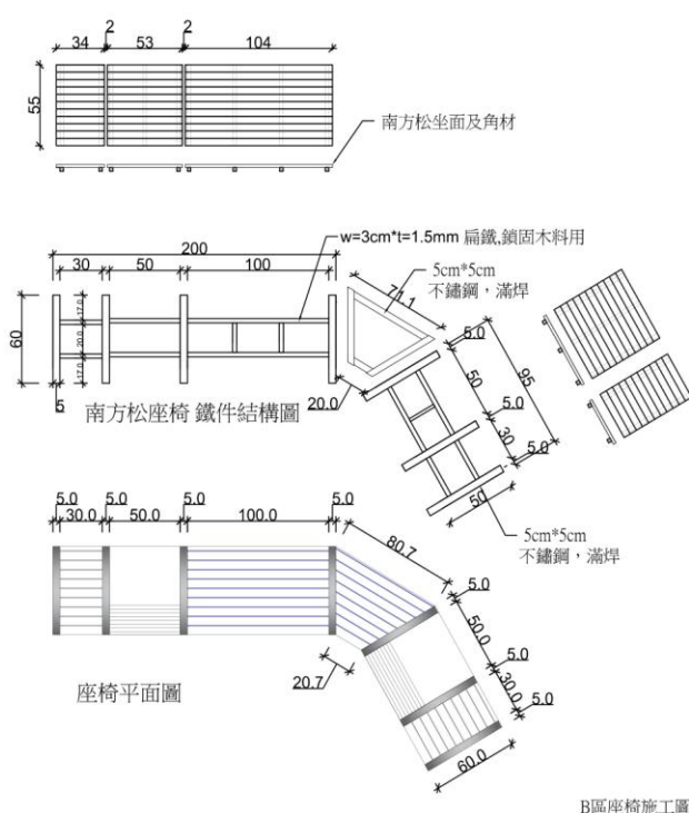
B區座椅施工圖
