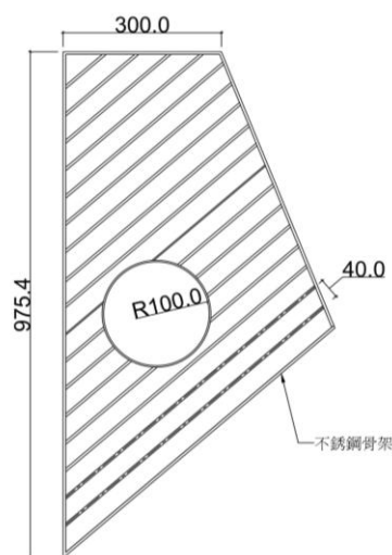
B區南方松平台 不銹鋼結構平面圖
