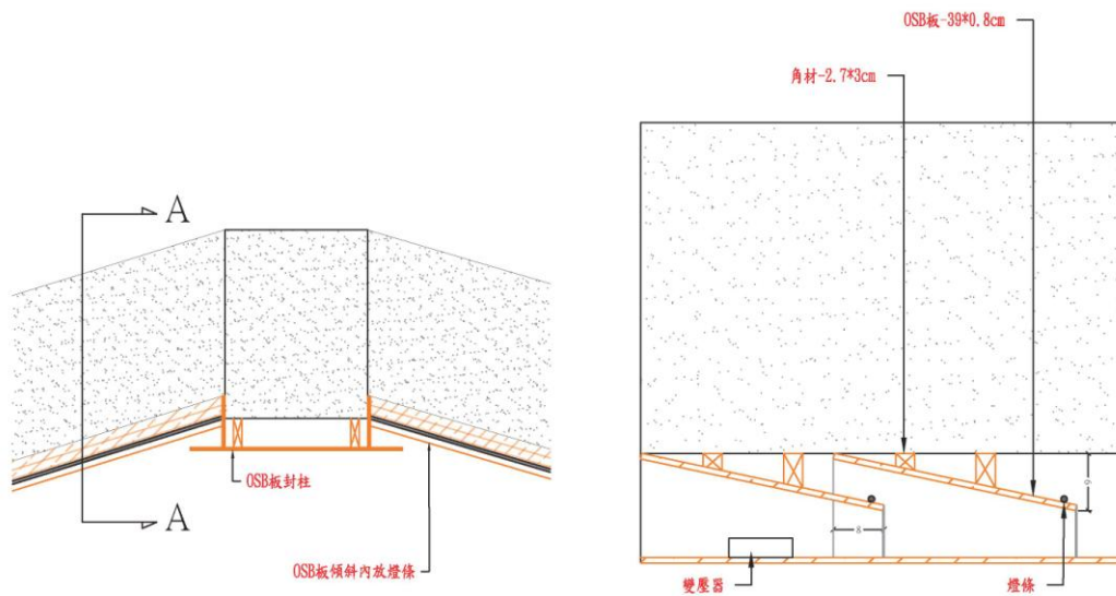
A-A剖面放大詳圖 2:1
