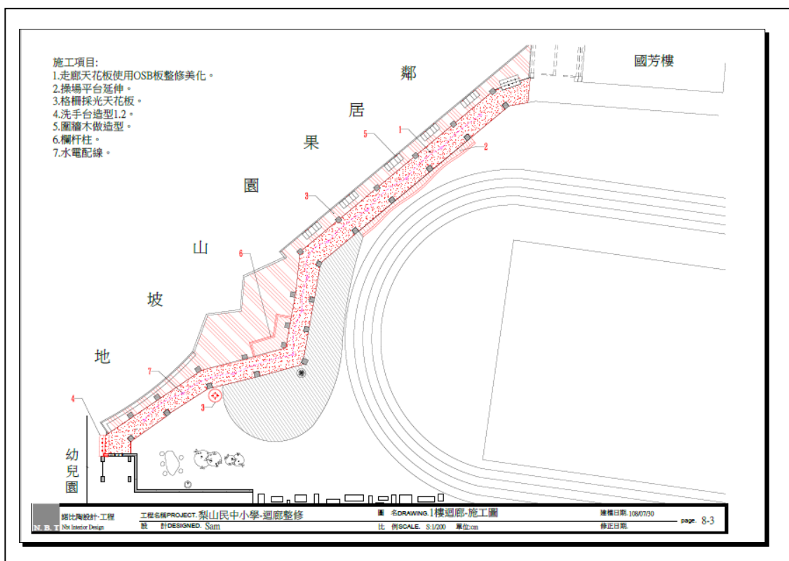
配置圖 B
