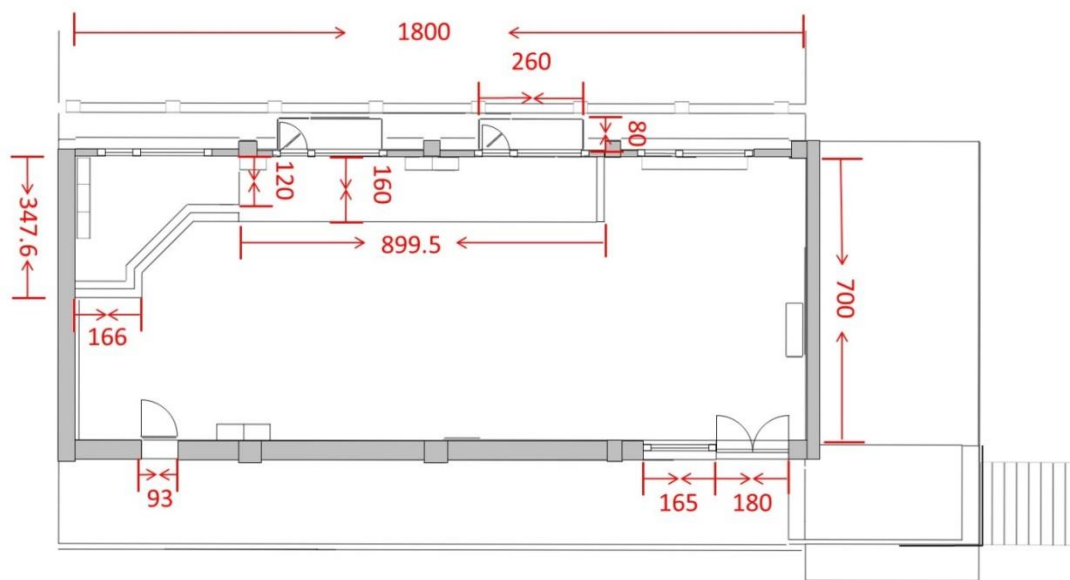
現況尺寸圖
