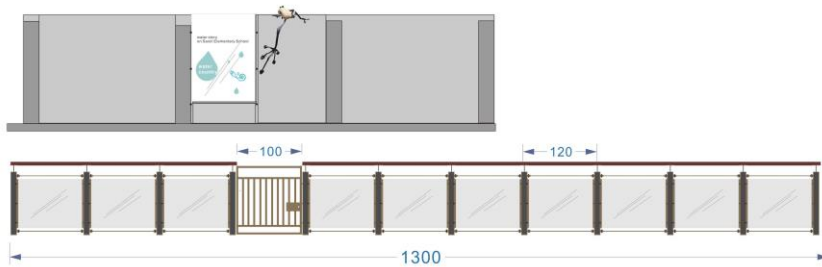
老牆及護欄竣工圖 (單位:cm)
