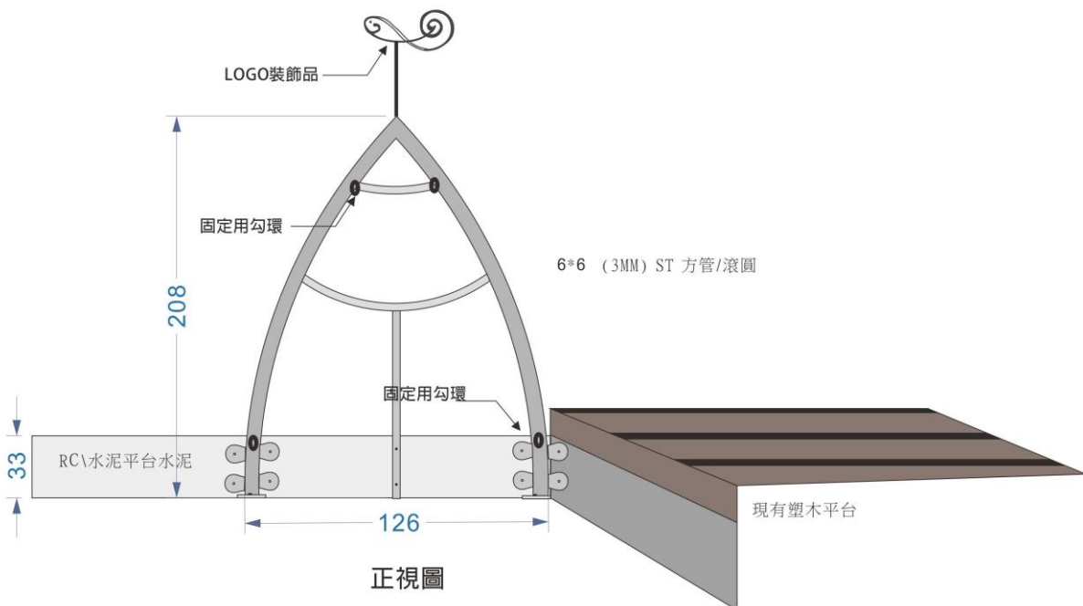
船架竣工圖
