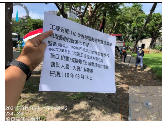
說明：鋪面基礎點焊鋼絲網鋪設
