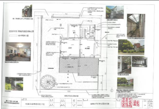
說明：1F 空間拆除位置
